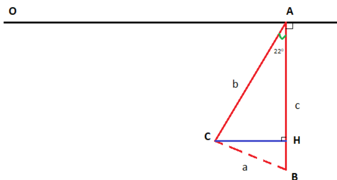
Att. 1: Risas dziļuma aprēķinu vizualizācija: AC – uz sāniem vērstais ultraskaņas vilnis, AB – uz leju vērstais ultraskaņas vilnis.
