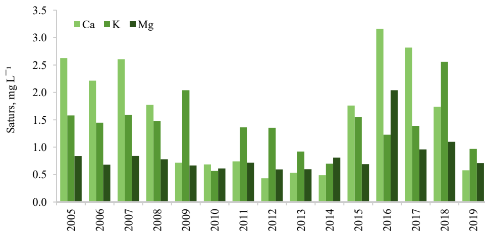
Att. 24: Bāzisko katjonu saturs augsnes ūdenī zem humusa slāņa laika posmā no 2004. līdz 2019. gadam Valgundes parauglaukumā.
