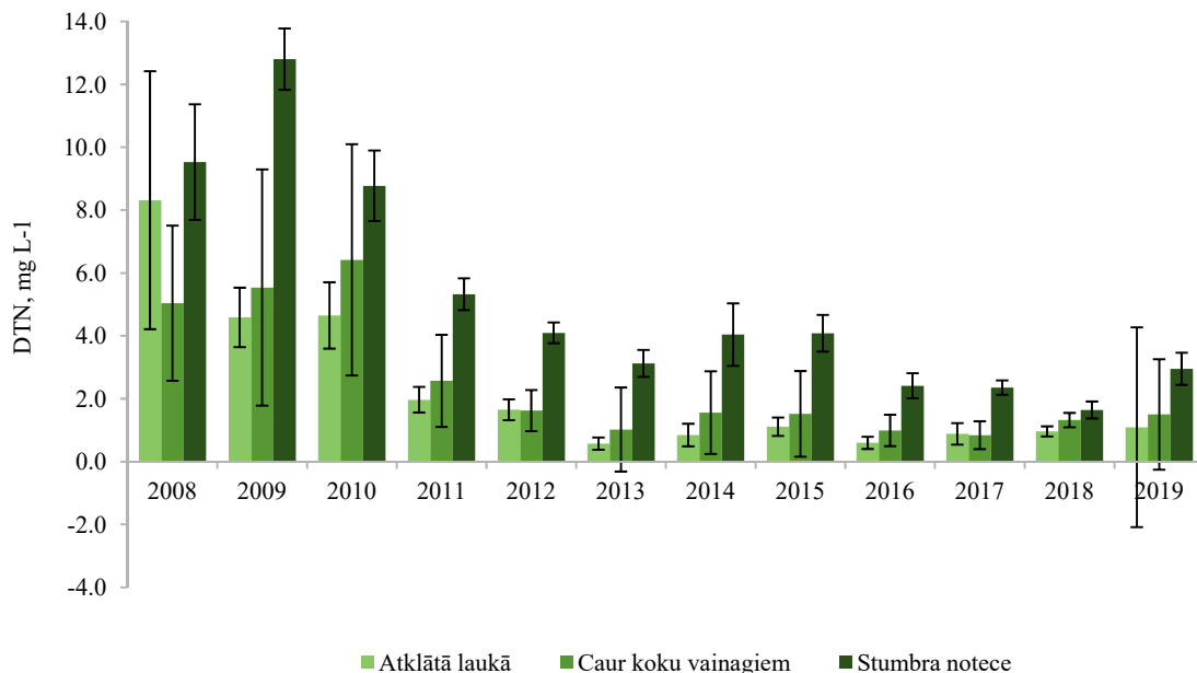
Att. 20: Vidējais kopējā slāpekļa (DTN) saturs nokrišņu ūdeņos Valgundes parauglaukumā kopš 2008. gada.
