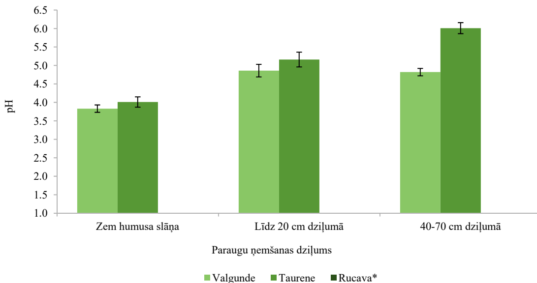
Att. 23: Augsnes ūdens vidējās pH vērtības Valgundes, Taurenes un Rucavas parauglaukumā 2019. gada novērojumu periodā; * - informācija nav pieejama, jo augsnes ūdens paraugu pieejamība bija ierobežota ilgstoša sausuma dēļ.
