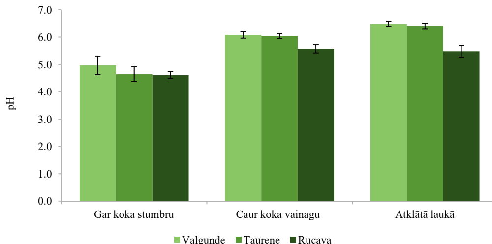
Att. 19: Vidējais nokrišņu ūdeņu pH Valgundes, Tauresnes un Rucavas parauglaukumos 2019. gadā.
