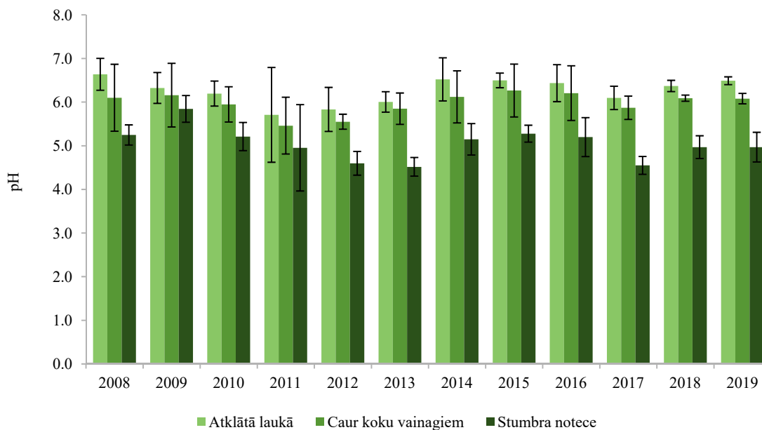
Att. 18: Atklātā lauka, koku vainagu caurteces un stumbru noteces nokrišņu vidējais pH laika posmā no 2008. līdz 2019. gadam Valgundes parauglaukumā.
