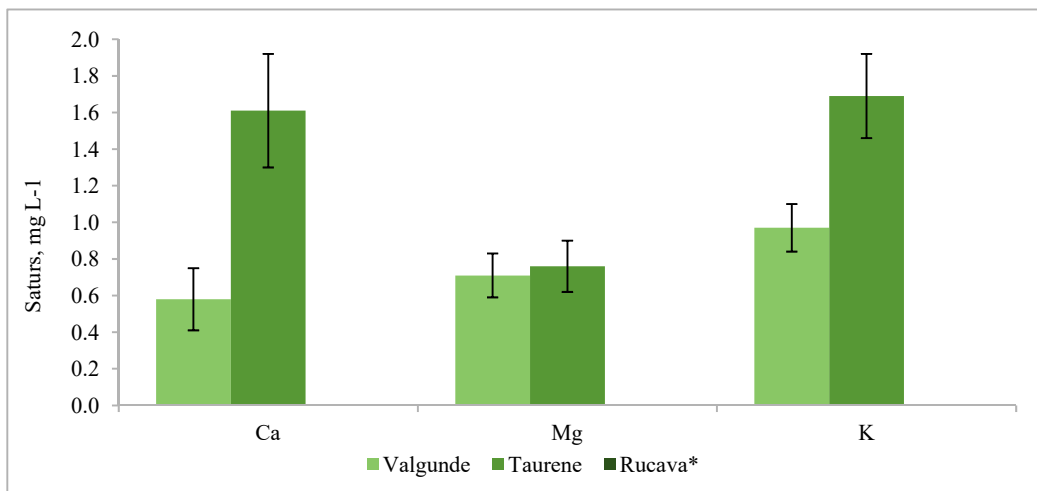
Att. 27: Bāzisko katjonu saturs augsnes ūdenī zem humusa slāņa 2019. gada novērojumu periodā Valgundes, Taurenes un Rucavas parauglaukumos; * - informācija nav pieejama, jo augsnes ūdens paraugu pieejamība bija ierobežota ilgstoša sausuma dēļ.
