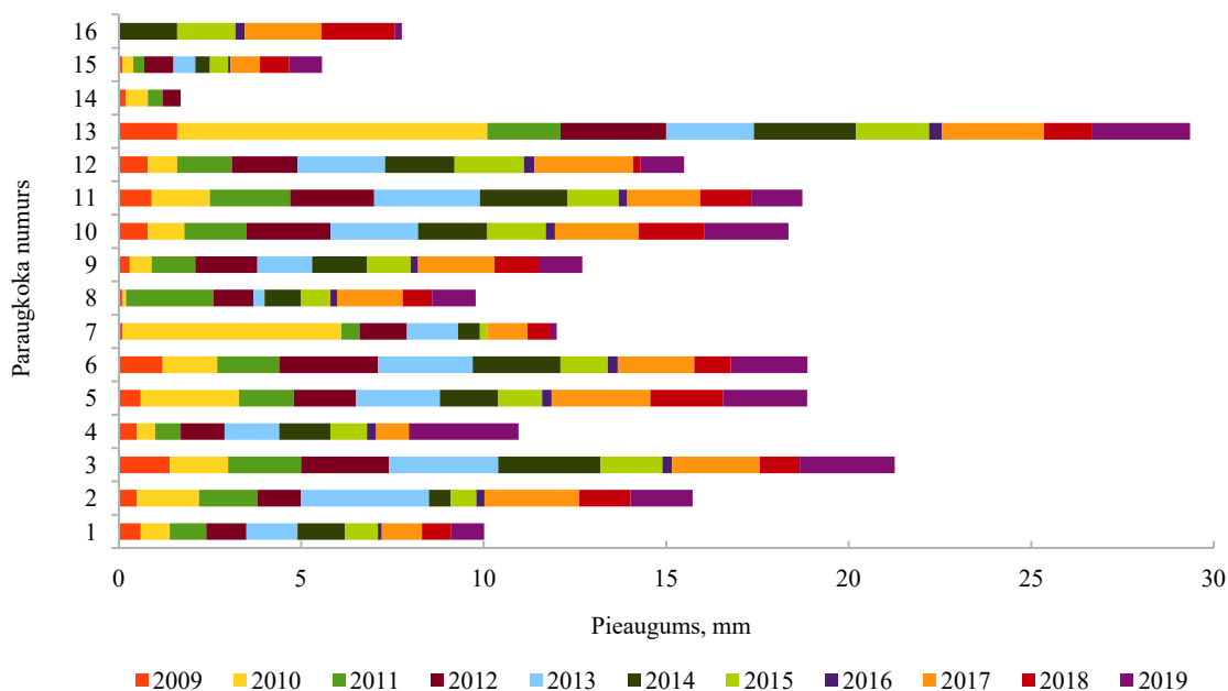
Att. 30: Koku pieauguma lentas mērījumi laika posmā no 2009. gada līdz 2019. gadam Valgundes parauglaukumā.
