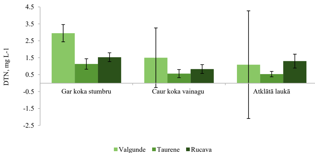
Att. 21: Vidējais kopējā slāpekļa (DTN) saturs nokrišņu ūdeņos Valgundes, Taurenē un Rucavas parauglaukumos 2019. gadā.
