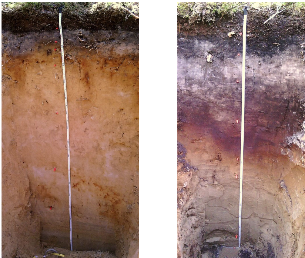
Att. 3: Augsnes profili Valgundes parauglaukumā, pa kreisi reljefa paaugstinājumā, pa labi reljefa pazeminājumā 4 .
