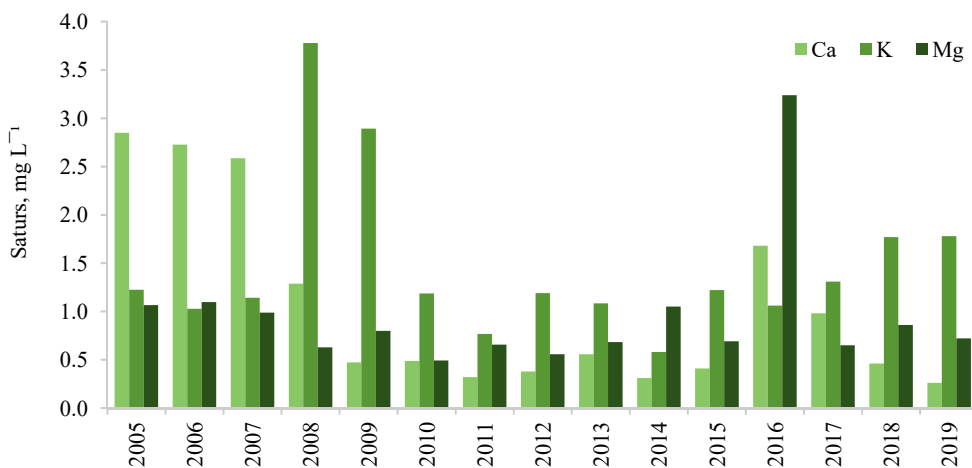
Att. 25: Bāzisko katjonu saturs augsnes ūdenī līdz 20 cm dziļumam laika posmā no 2004. līdz 2019. gadam Valgundes parauglaukumā.
