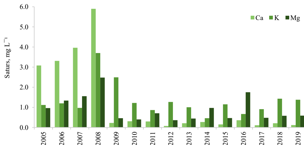
Att. 26: Bāzisko katjonu saturs augsnes ūdenos 40-70 cm dziļumā laika posmā no 2004. līdz 2019. gadam Valgundes parauglaukumā.
