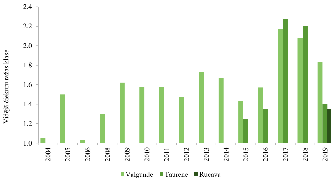
Att. 12: Čiekuru raža Valgundes, Taurenes un Rucavas parauglaukumā.
