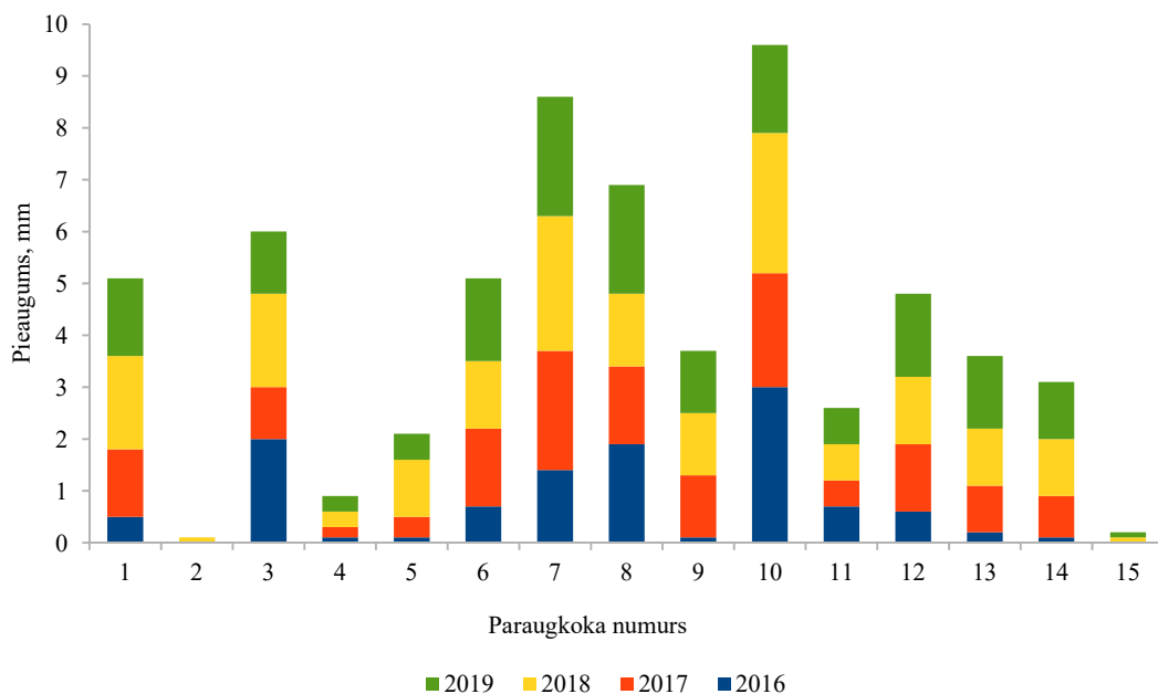
Att. 31: Koku pieauguma lentas mērījumi laika posmā no 2016. gada līdz 2019. gadam Taurenes parauglaukumā.
