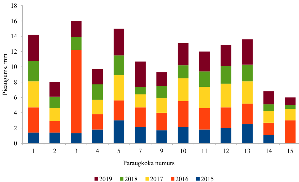
Att. 32: Koku pieauguma lentas mērījumi laika posmā no 2015. gada līdz 2019. gadam Rucavas parauglaukumā.
