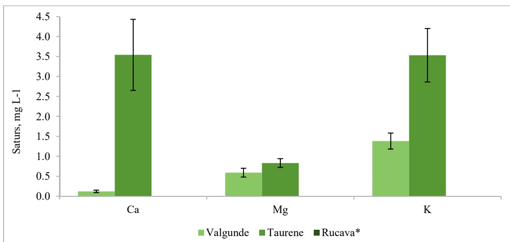
Att. 29: Bāzisko katjonu saturs augsnes ūdenī 40-70 cm dziļumā 2019. gada novērojumu periodā Valgundes, Taurenes un Rucavas parauglaukumos; * - informācija nav pieejama, jo augsnes ūdens paraugu pieejamība bija ierobežota ilgstoša sausuma dēļ.
