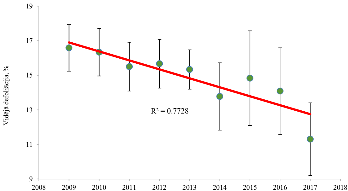
Att. 11: Koku vainagu vidējā defoliācijas dinamika Valgundes parauglaukumā laika posmā no 2009. gada līdz 2017. gadam.
