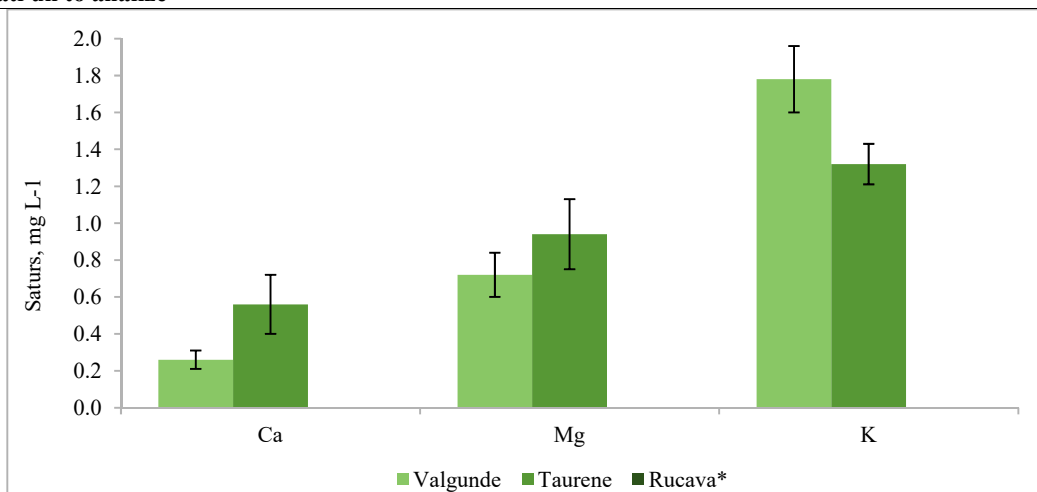
Att. 28: Bāzisko katjonu saturs augsnes ūdenī līdz 20 cm dziļumam 2019. gada novērojumu periodā Valgundes, Taurenes un Rucavas parauglaukumos; * - informācija nav pieejama, jo augsnes ūdens paraugu pieejamība bija ierobežota ilgstoša sausuma dēļ.
