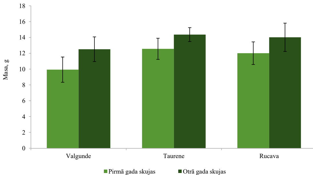
Att. 15: Pirmā un otrā gada pieauguma 1000 skuju vidējā masa Valgundes, Taurenes un Rucavas parauglaukumos 2017. gadā.
