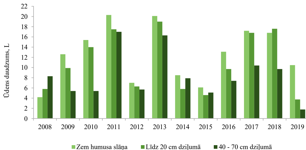
Att. 17: Augšnes ūdeņu daudzuma izmaiņas no 2008. līdz 2019. gadam Valgundes parauglaukumā.
