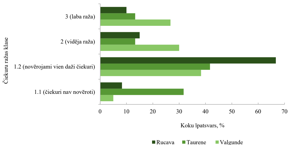
Att. 13: Čiekuru ražas salīdzinājums Valgundes, Taurenes un Rucavas parauglaukumos 2019. gadā.
